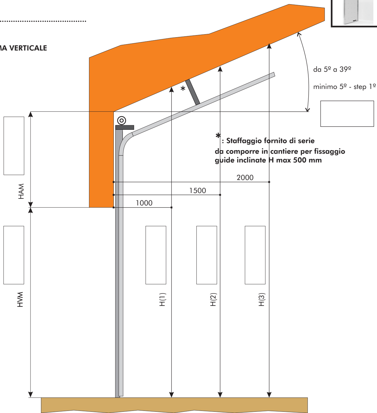
SCHEMA ORIZZONTALE
